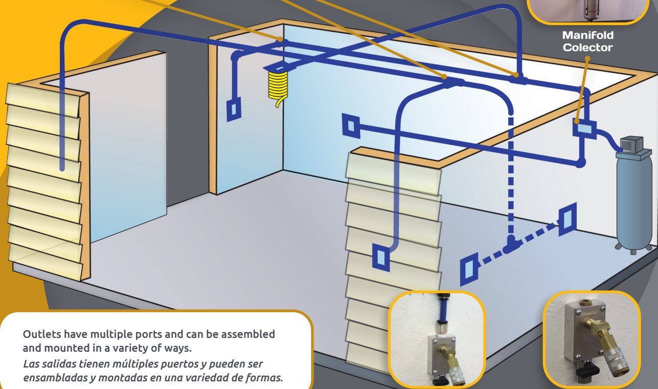
Surface Mount Montaje en Superficie Air line is mounted to wall La línea de aire está montada en la pared
