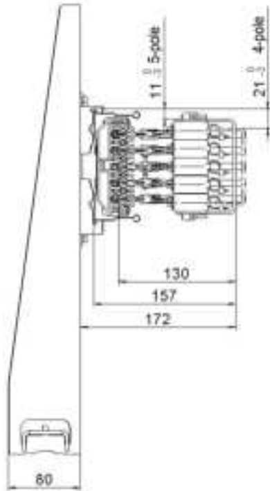
Fig. 83: Current collector 0831 (Order No.: 083103-...)
