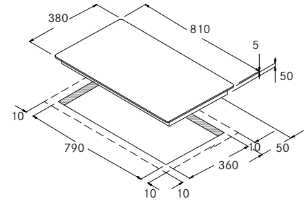
3 PIN SUPER STRETTA
