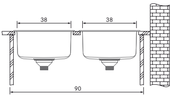
RAX-610-38 montaje doble en mueble de 90 cm.
