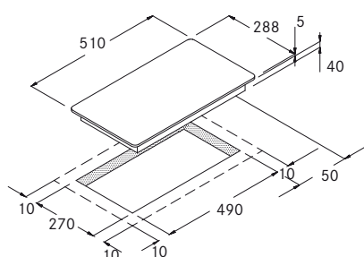
Vitro TX-302, Vitro IX-302
