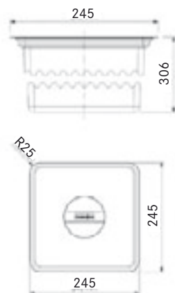
WASTE-BIN K10 CUA
