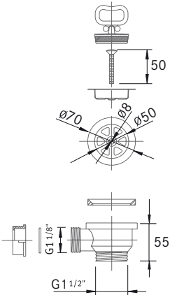
Válvula "A"
