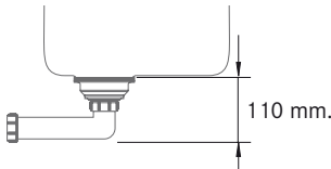
Distancia ocupada por debajo del fregadero Válvulas (A, B, BG, C, D y DG) + codo del Sifón (SF1, SF2)
