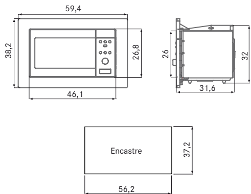
MICROONDAS TECH 17G
