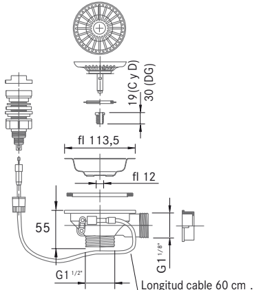
Válvula "C" / "D" / "DG"
