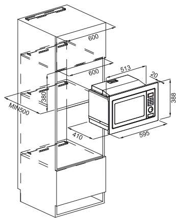
MICROONDAS CRYSTAL 250 SMART 250
