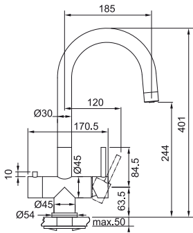
EOS CLEAR INOX (3 vías)
