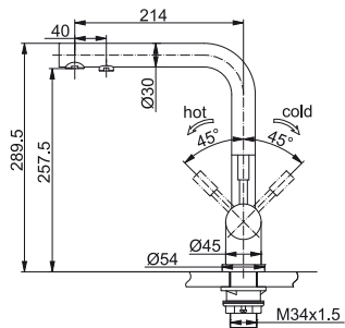
ATLAS CLEAR INOX (3 vías)
