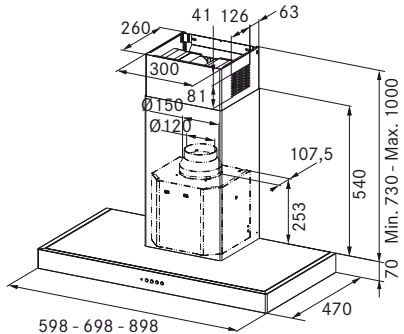
ITALIA 60 ITALIA 70 ITALIA 90
