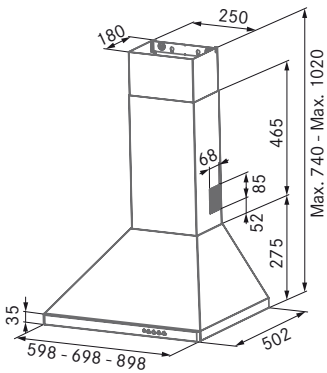
D'ECO 60 D'ECO 70 D'ECO 90
