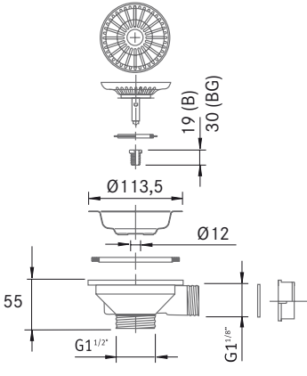
Válvula "B" / "BG"
