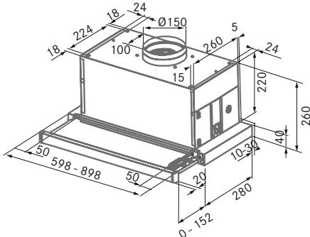
MEGA FLEX 60 MEGA FLEX 90
