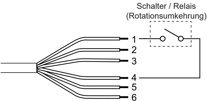
LEGENDE SIGNALKABEL
