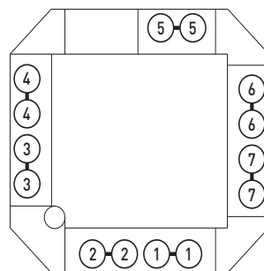
Schéma de raccordement
