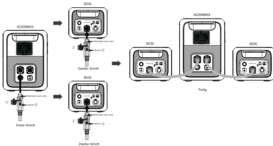
Abbildung: Kapazitätserweitertes Modus der BLUETTI AC200MAX
