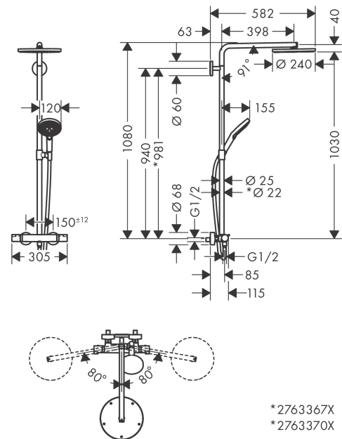
Maßzeichnung
