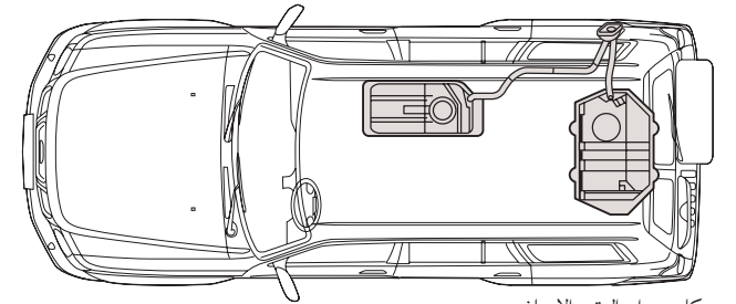
مكان خزان الوقود الإضافي Sub-fuel tank location
