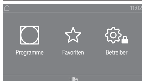
Hauptmenü
