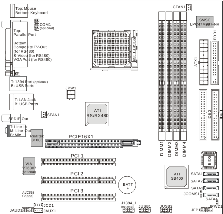
RS480M2/RX480M2 (MS-7093 v1.X) M-ATX Mainboard
