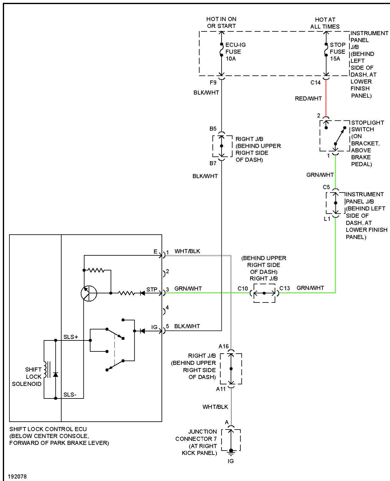
Fig. 37: Shift Interlock Circuit
