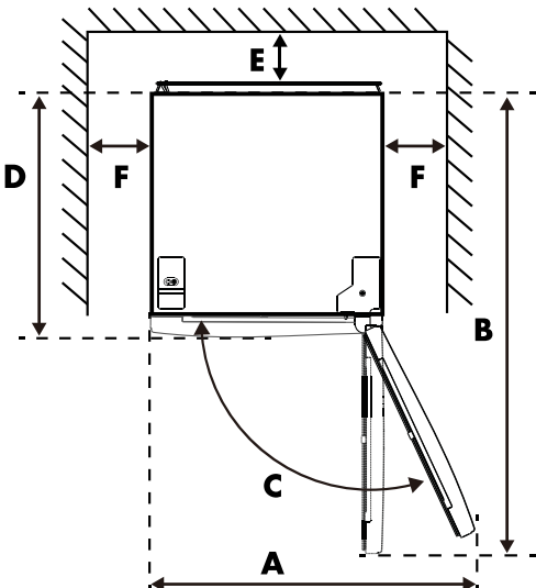
• Abbildung 2. Draufsicht
