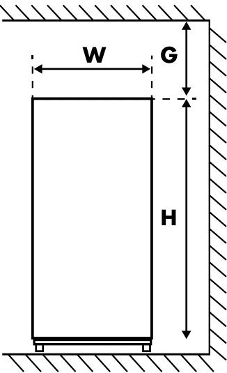
• Abbildung 1. Vorderansicht
