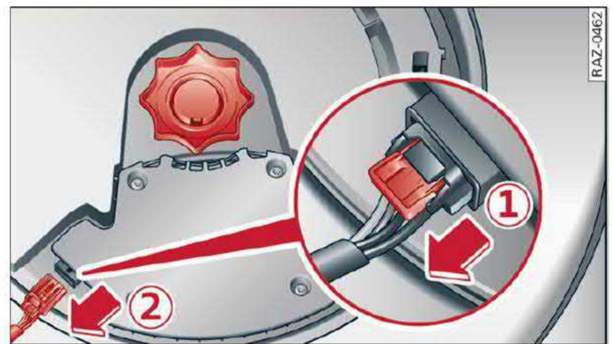
Fig. 164 Spare tire well: subwoofer
