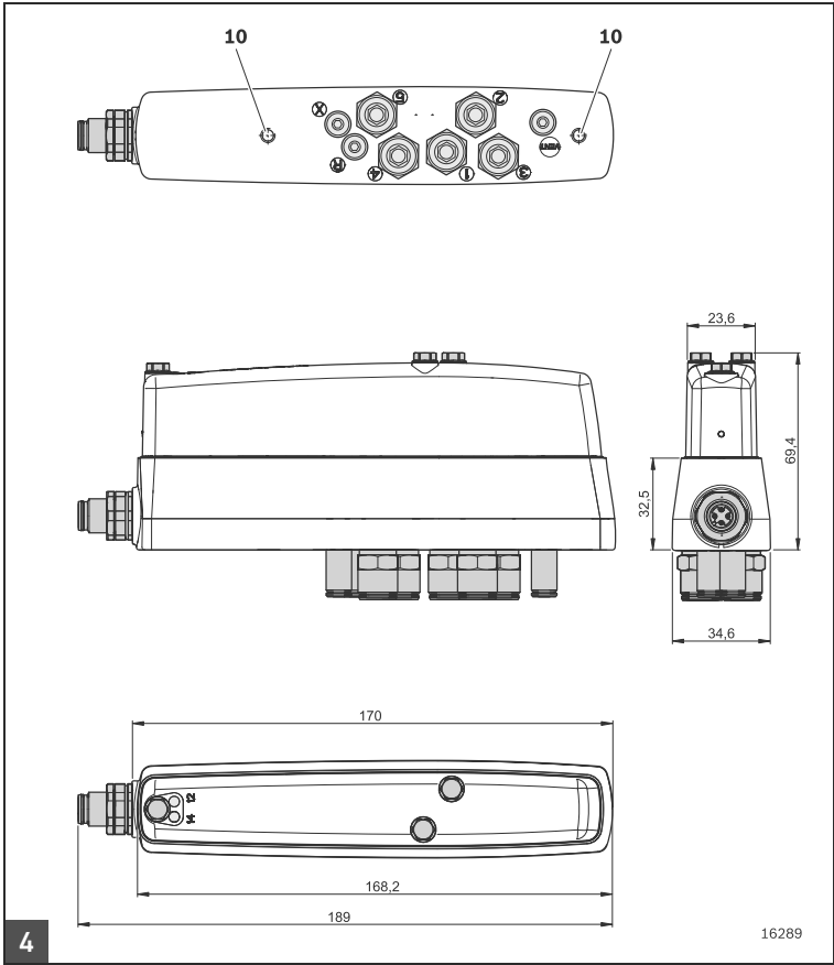
Montaggio della valvola singola CL03 con piastra base e valvola - Disegno quotato Montaje de la válvula individual CL03 con placa base y válvula: Esquema acotado Montera singelventil CL03 med basplatta och ventil - Måttitning
