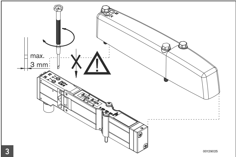
Azionamento manuale / Accionamiento auxiliar manual / Manuell omställning
