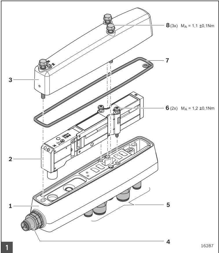
Panoramica valvola singola CL03 con piastra base e copertura valvola Vista general de la válvula individual CL03 con placa base y cubierta de válvula Översikt singelventil CL03 med basplatta och skyddskåpa
