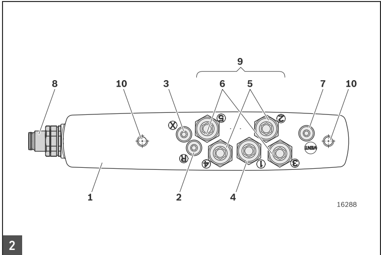
Panoramica piastra base / Vista general de la placa base / Översikt basplatta
