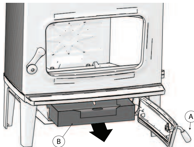
Fig. 14 Cajón cenicero
