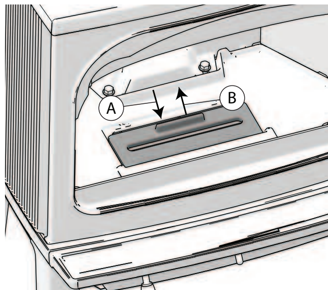
Fig. 13 Rejilla
