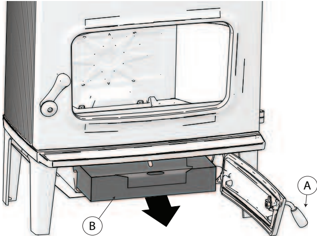
Fig. 16 Ash pan
