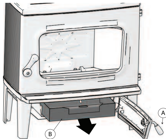
Fig. 14 Cassetto ceneraio
