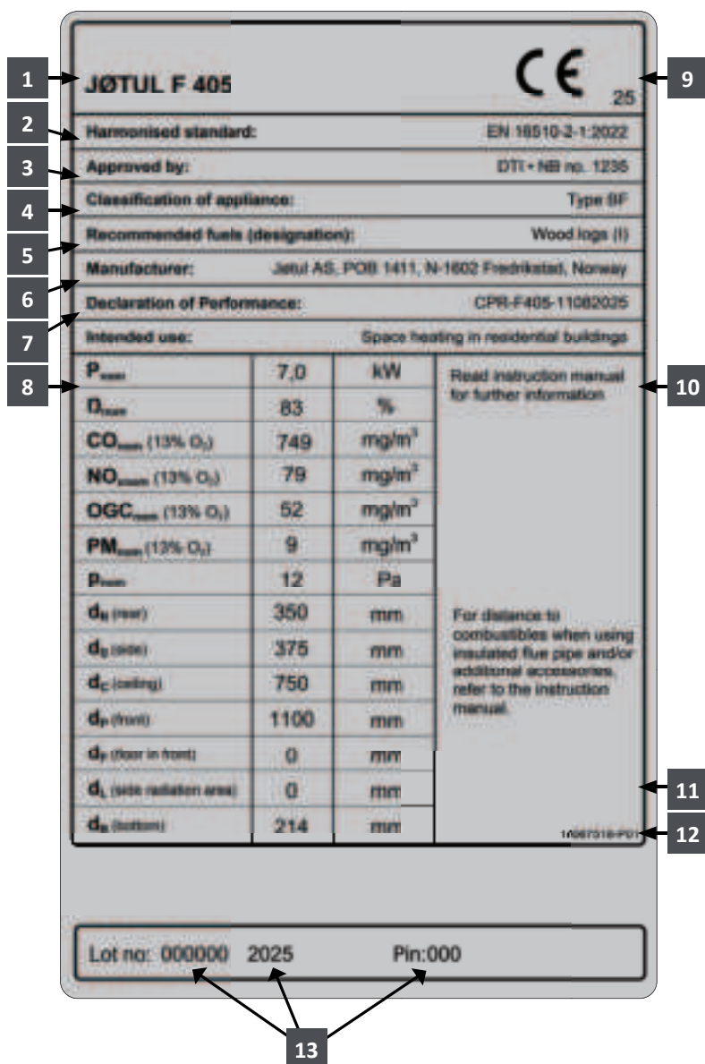
Plaque signalétique
