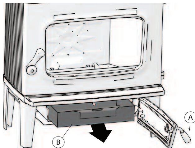
Fig. 14 Cendrier
