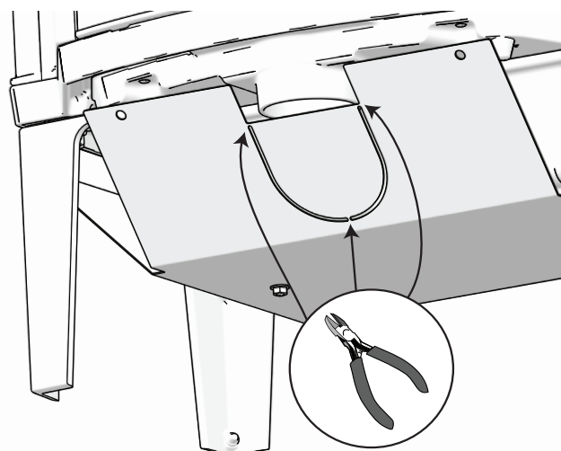
Fig. 8 Montage du raccord d'arrivée d'air frais
