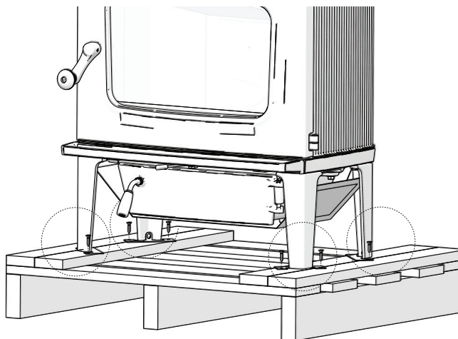
Fig. 2 Dépose de la palette
