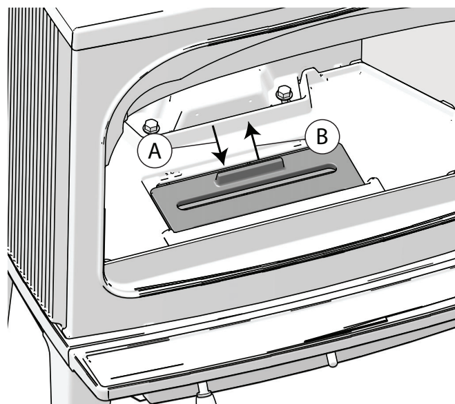
Fig. 13 Rejilla
