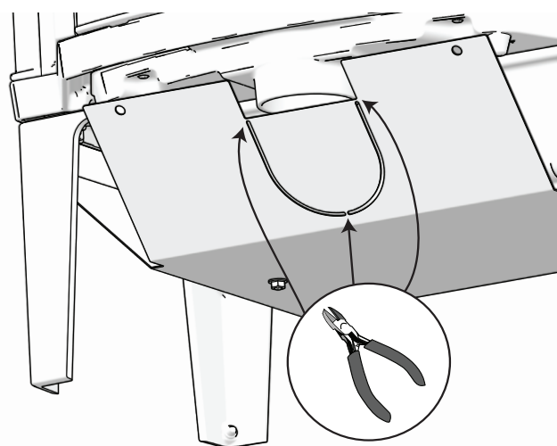
Fig. 8a Montare il collegamento di alimentazione dell'aria esterna
