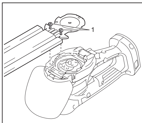
► 1. Screws
