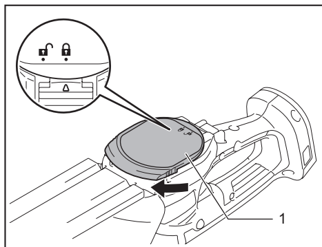
► 1. Undercover
