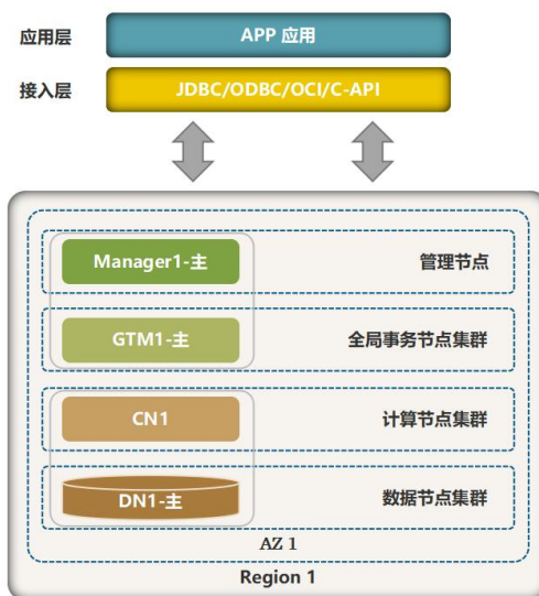
图 3.3-1 单管理节点组网图
