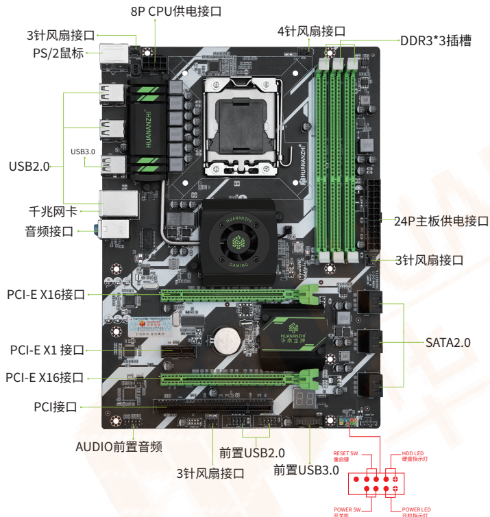
图1-1 X58至尊主板图解
