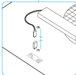
Fig. 3 Enkel montering av mottakeren. Mottakeren kan monteres enkelt uten behov for verktøy. Fjern USB-pluggen (1) fra viftens overside, og plugg inn mottakeren (3).
