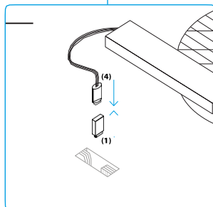
Fig. 3 Enkel montering av mottagaren. Mottagaren installeras lätt utan behov av extra verktyg. Avlägsna stiftet (1) på spiskåpens överdel och för in mottagaren (4).
