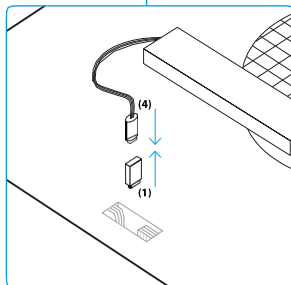
Fig. 3 Montage facile du récepteur, il est possible d'installer facilement le récepteur sans outil supplémentaire : Retirez le stick de la partie supérieure de la hotte aspirante (1) en insérant le récepteur (4).
