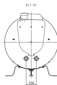
OKC 80–125 NTR/Z
