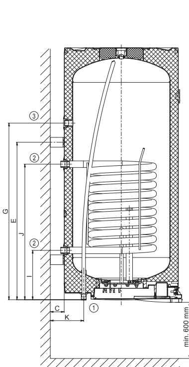
OKC 160–200 NTR/Z
