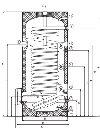
OKC 200 NTR/HP
