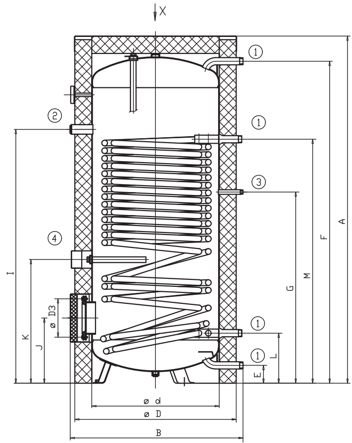
OKC 750, 1000 NTR/HP
