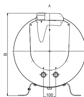
OKC 160–200 NTR/Z
