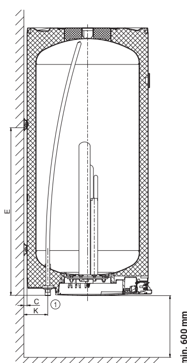
OKCE 200 2/6 (4) kW
