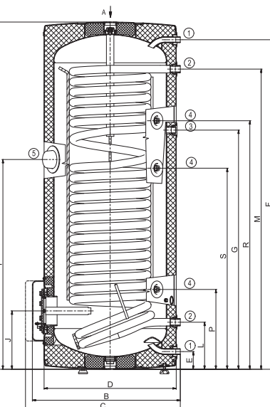
OKC 250 NTR/HP
