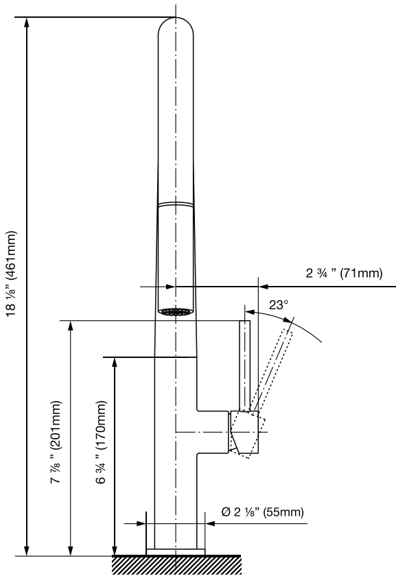
SIDE VIEW / VUE DE CÔTÉ / VISTA LATERAL
