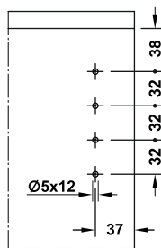
Drilling pattern for cabinet ระยะเจาะสำหรับตู้
