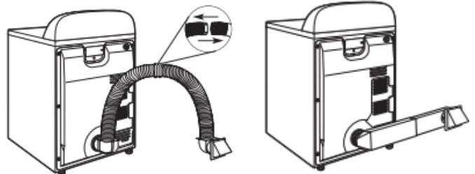
Installation au-dessus de la sécheuse Installation en pénétration par le mur (également offerte avec un coude décalé)
