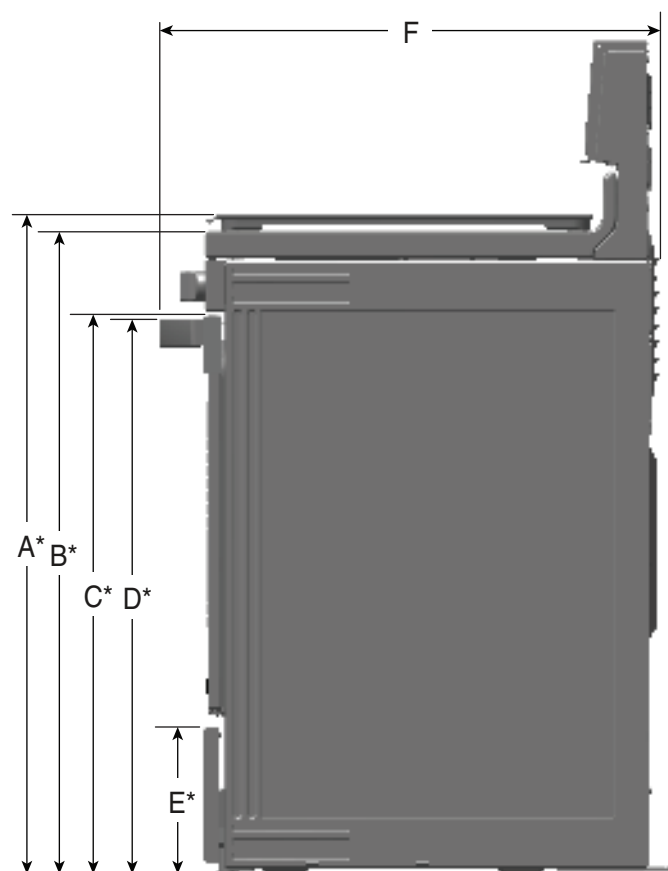
VUE LATÉRALE
