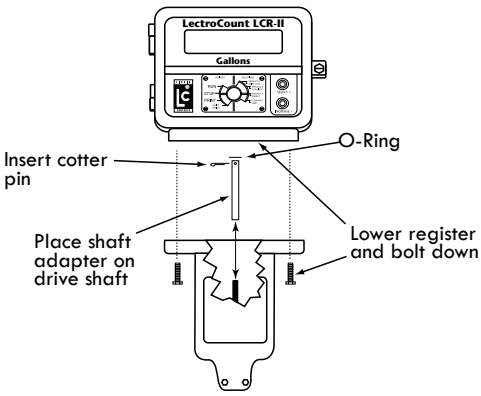
LC Meter
