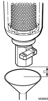
Fig. 1. Drenaje del agua de enjuague.
