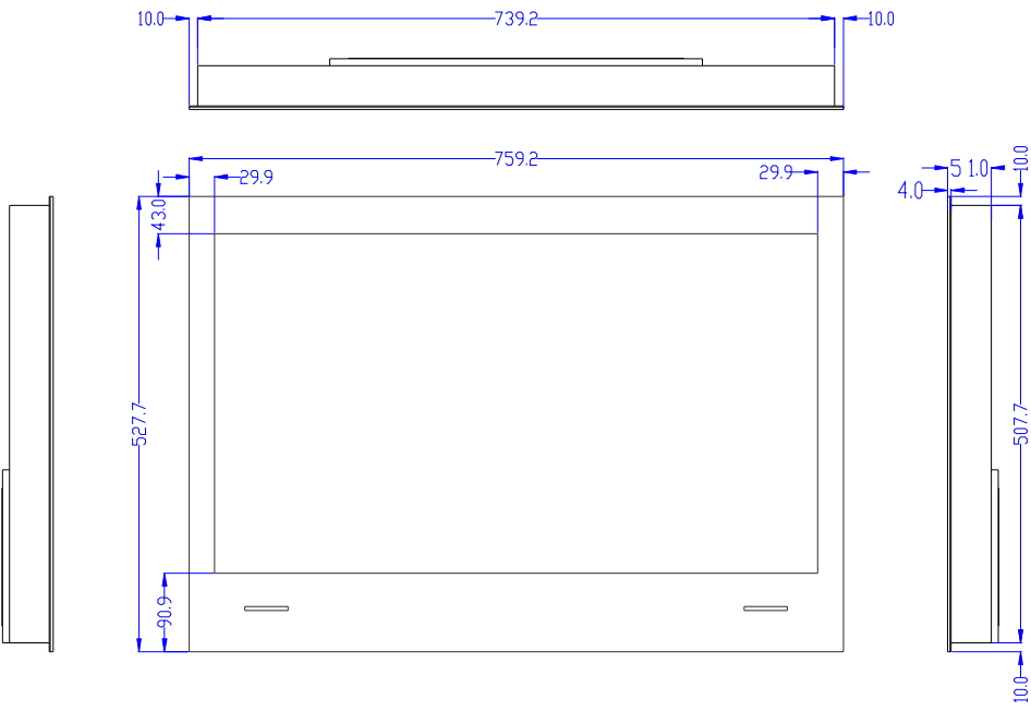
Television(Unit:mm)
