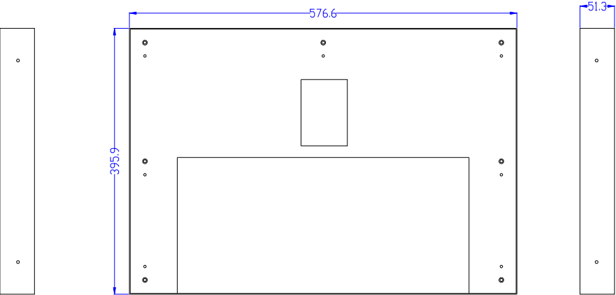
Bracket(Unit:mm)
