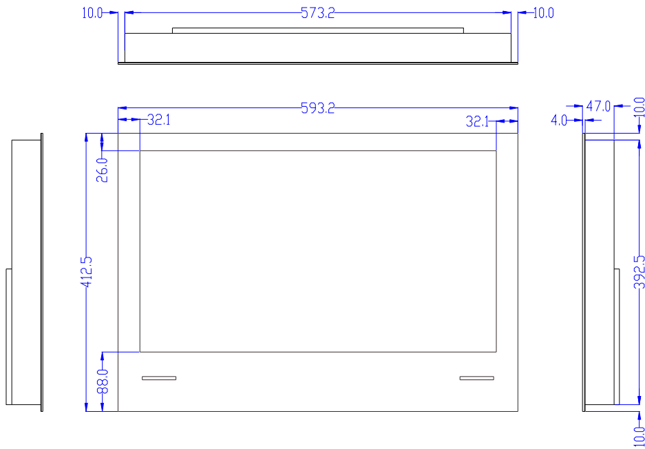
Television(Unit:mm)
