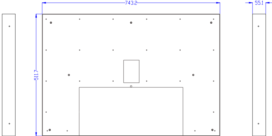
Bracket(Unit:mm)
