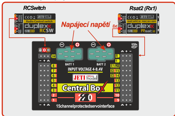
Obr. 4: Aplikační zapojení s RCSwitchem
