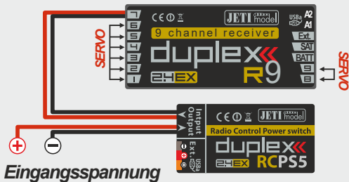
Bild 5: Anschlussbeispiel mit RCPower Switch
