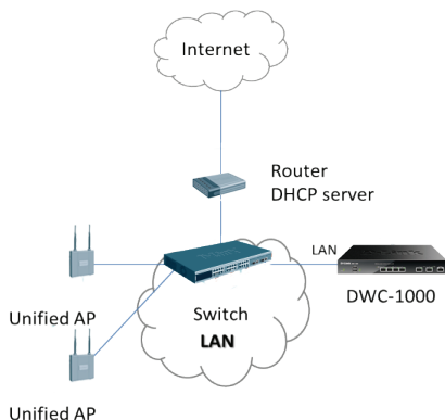
Figura 8. Esempio di distribuzione della rete WLAN
