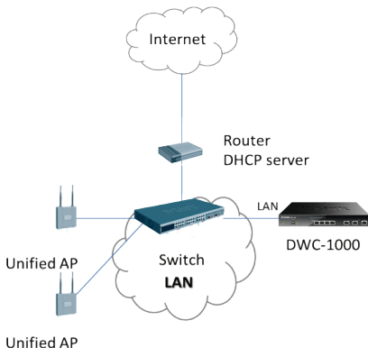
Abbildung 8. Beispiel einer WLAN-Installation
