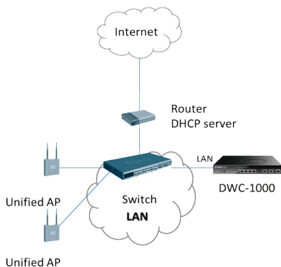
Figure 8. Exemple de déploiement d'un réseau local sans fil
