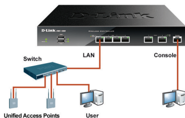
Figure 5. Exemple de connexion de base
