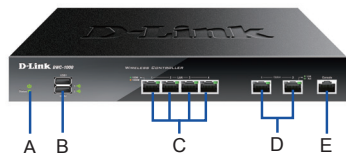
Abbildung 1. Vorderseite des DWC-1000
