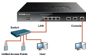
Figura 5. Esempio di collegamento di base
