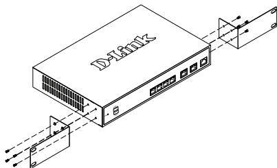
Figura 3. Acople los soportes de montaje en estante
