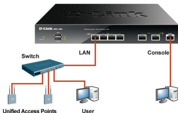
Figura 5. Ejemplo de conexión básica
