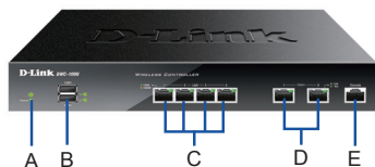
Figura 1. Pannello frontale del dispositivo DWC-1000
