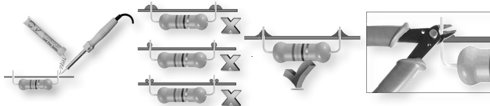
Component side - Componentenzijde - Côte composants - Bauteileseite - Lado de los componentes
