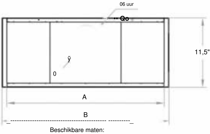
BOVENAANZICHT
