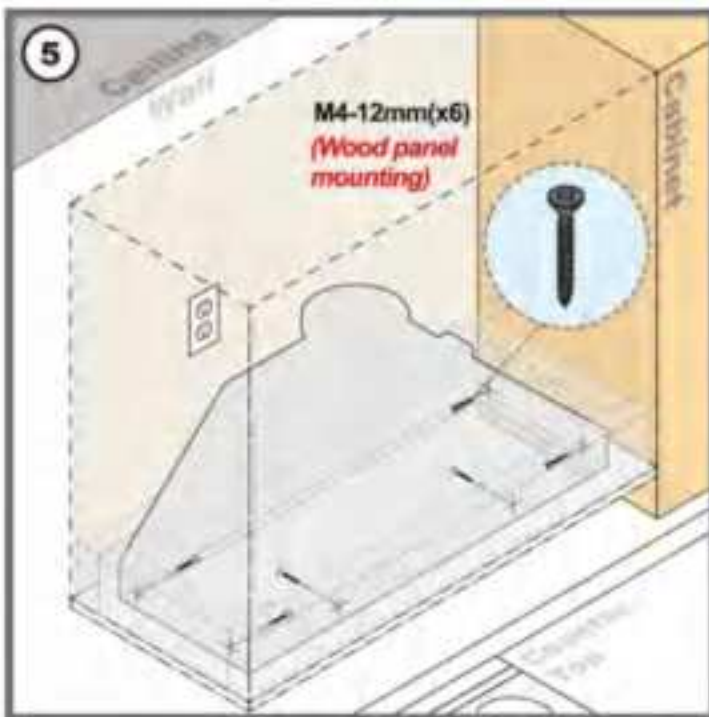
(5) Die restlichen Schrauben von der Innenseite der Dunstabzugshaube aus am Holzklötz befestigen.
