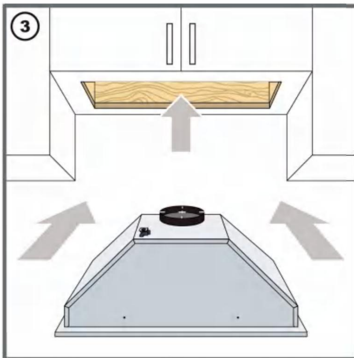
(3) Plaats en schuif de afzuigkap voorzichtig in het bovenkastje.
