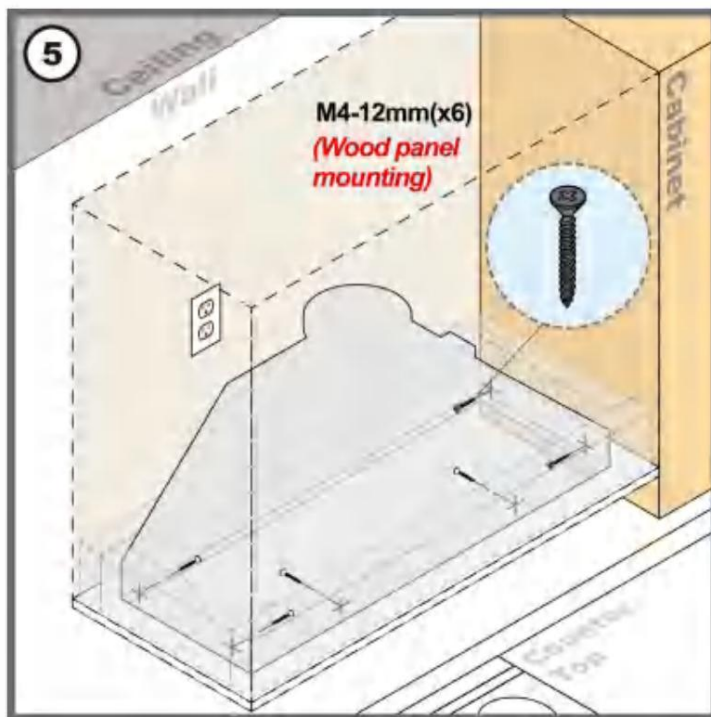
(5) Fije los tornillos restantes desde el lado interior de la campana extractora al bloque de madera.
