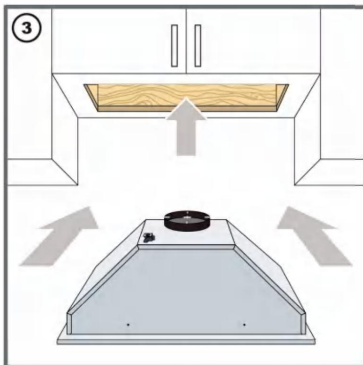
(3) Sätt försiktigt in och skjut spiskåpan i överskåpet.
