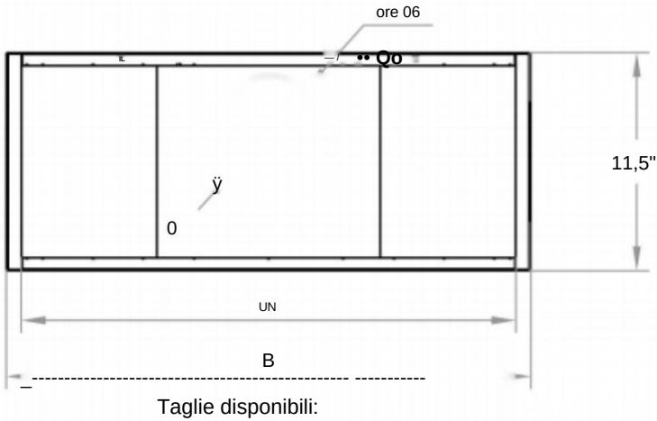
VISTA DALL'ALTO
