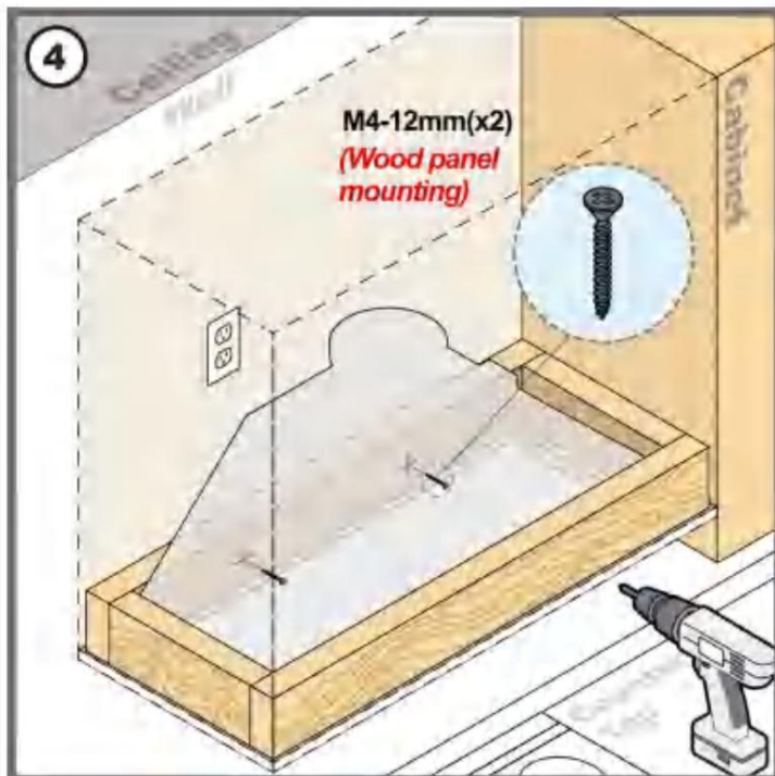
(4) Bevestig de afzuigkap via de montagegaten met houtschroeven aan de houten blokkering.
