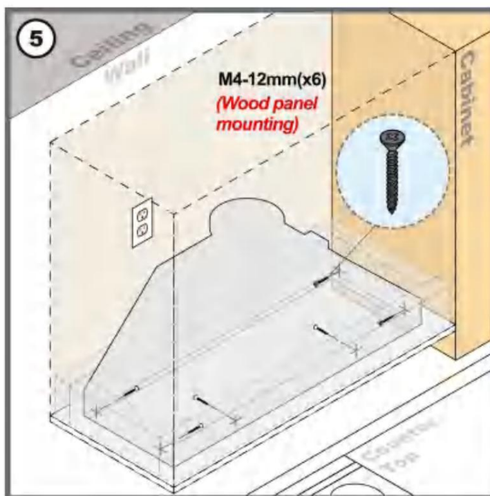
(5) Fissare le viti rimanenti dal lato interno della cappa al blocco di legno.
