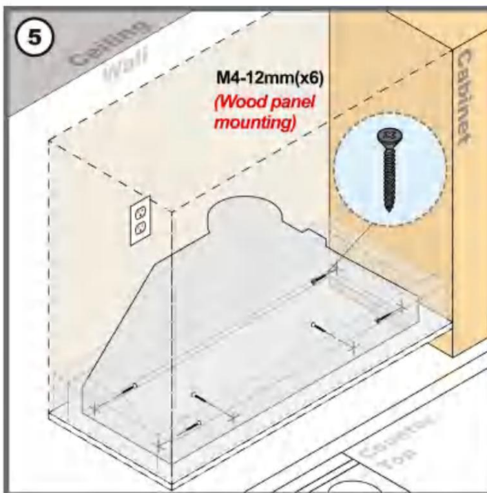
(5) Bevestig de resterende schroeven aan de binnenkant van de afzuigkap aan de houten blokkering.
