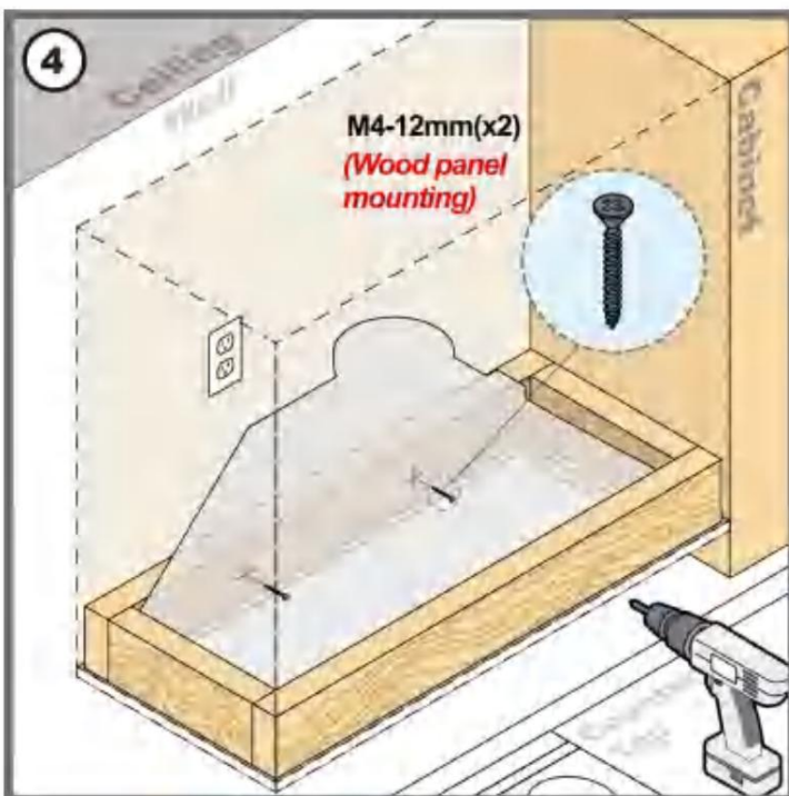
(4) A través de los orificios de instalación, fije la campana extractora con tornillos para madera para montarla sobre el bloque de madera.
