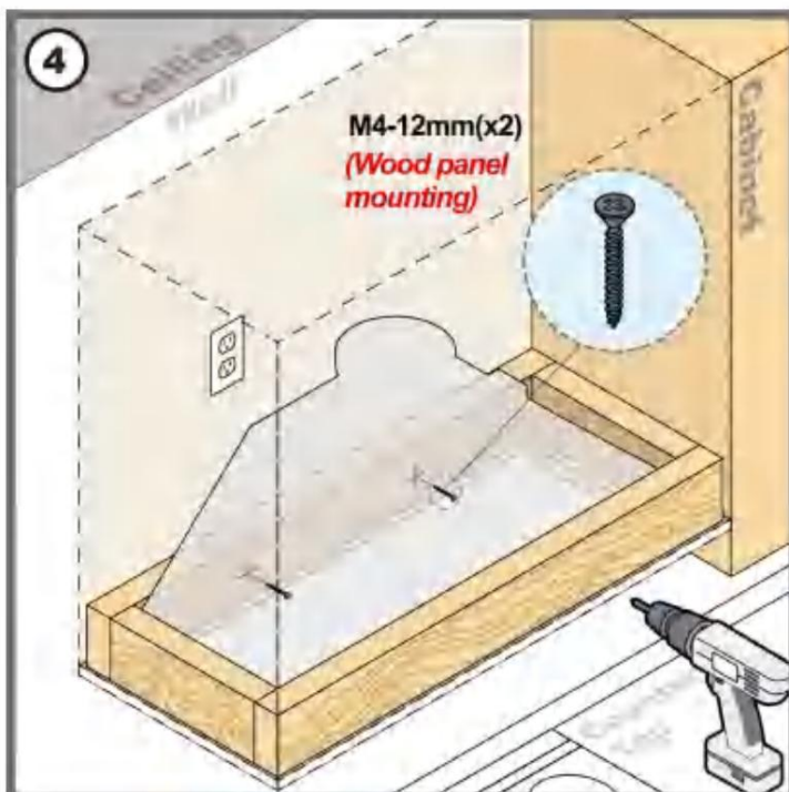
(4) Die Dunstabzugshaube durch die Montagelöcher führen und mit Holzschrauben auf dem Holzklotz befestigen.
