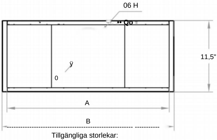
TOPPVISNING
