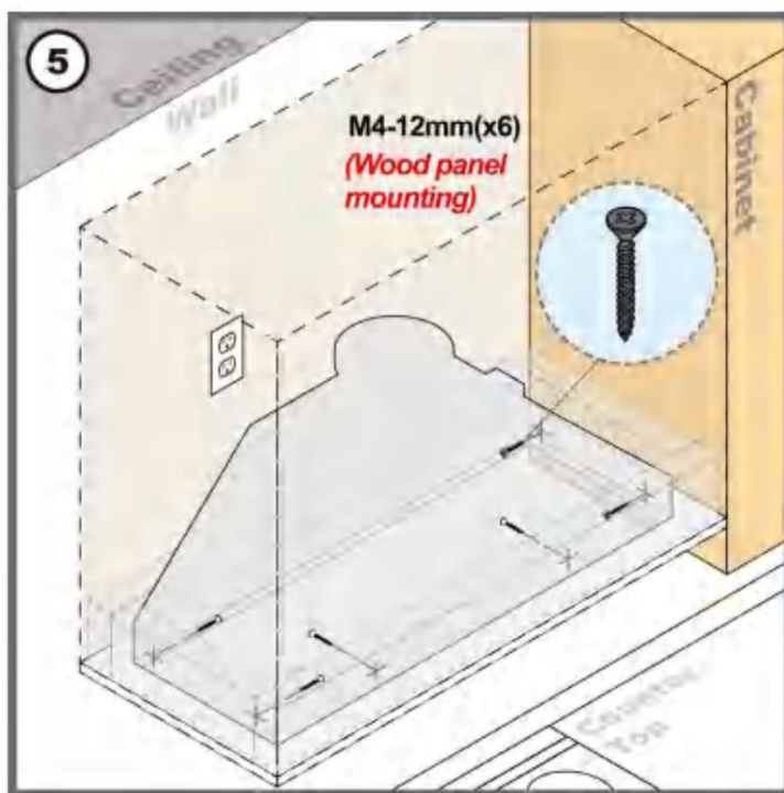
(5) Przykręć pozostałe śruby od wewnętrznej strony okapu do blokady drewnianej.
