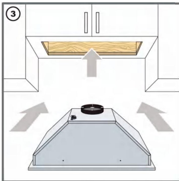
(3) Inserire e far scorrere con attenzione la cappa nel mobiletto superiore.
