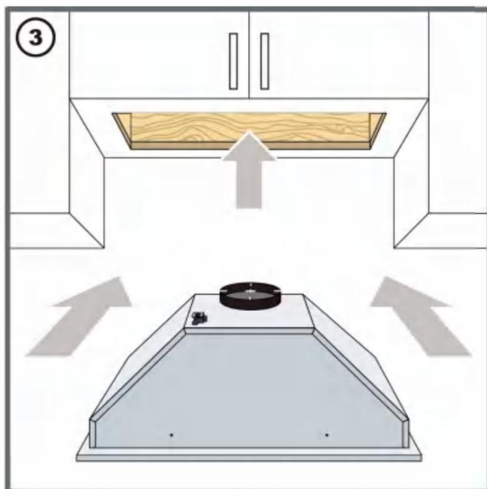
(3) Ostrożnie wsuń okap kuchenny do szafki górnej.
