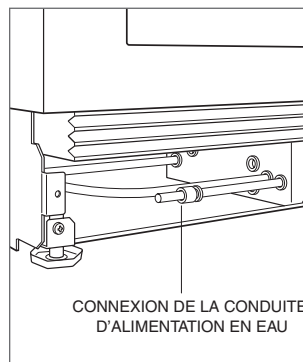
Connexion de la conduite d'alimentation en eau
