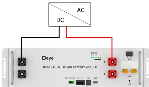
Abbildung 5-2: Einzelbatterieanschluss
