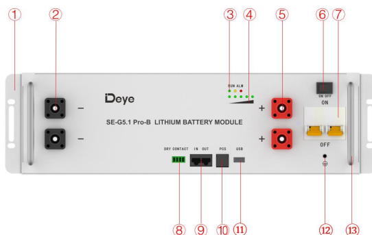
Abbildung 2-1: Das vordere Bedienfeld
