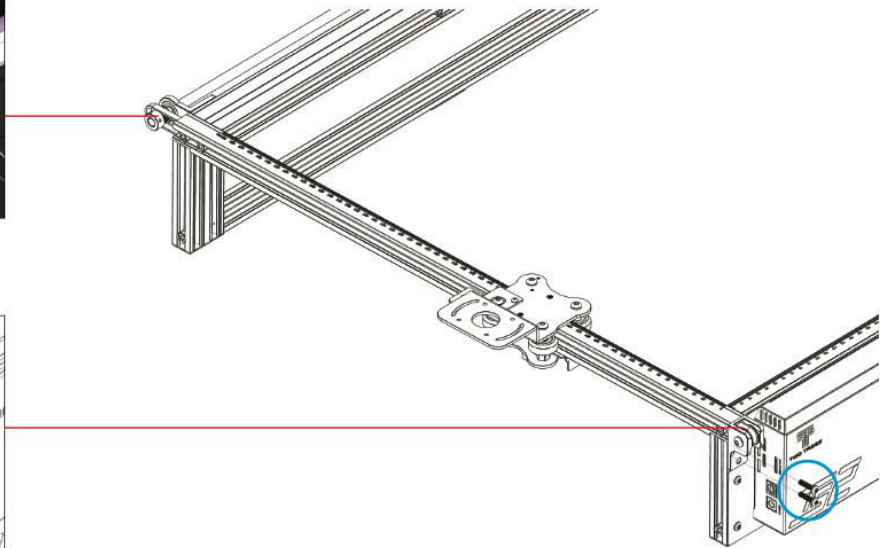
Synchrones Rad
