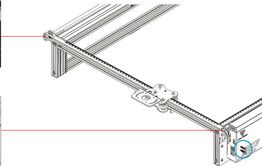
Synchronní kolo
