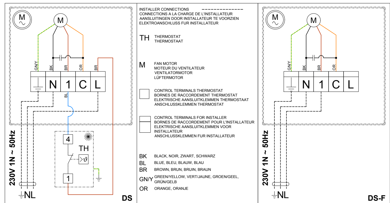
Abbildung 3 Interner Schaltplan
