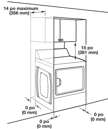
Installation dans un encastrement
