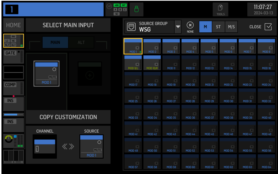
Fig. 6: SOURCE GROUP WSG をチャンネルに割り当てる
