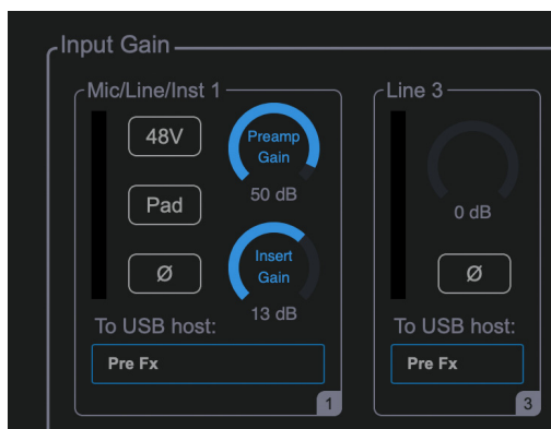
Figura 4-3. Se producen 54 dB de ganancia antes del punto de inserto, mientras que después se producen 20 dB. Juntos, proporcionan hasta 74 dB de ganancia.
