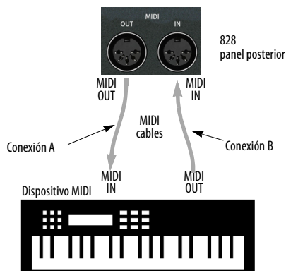
Figura 4-5. Conexión de un dispositivo MIDI a la 828.
