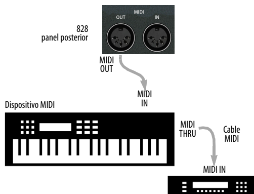
Figura 4-6. Conexión de dispositivos adicionales con puertos MIDI THRU.
