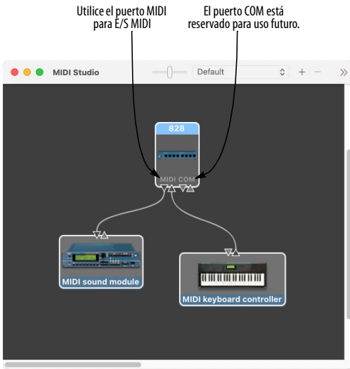
Figura 3-2. Conexión de dispositivos a la 828. En este ejemplo, se conecta un teclado controlador al MIDI IN de la 828 y un módulo de sonido a la 828 MIDI OUT.
