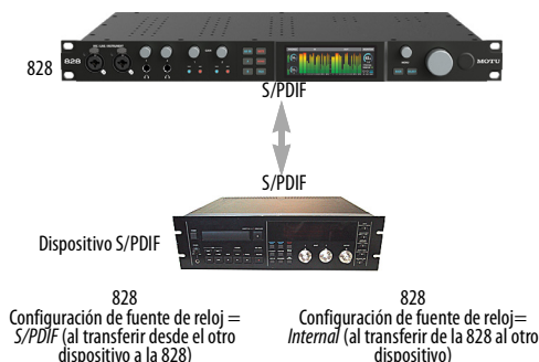
Figura 4-10. La configuración para sincronizar un dispositivo S/PDIF con la 828. La sincronización se logra a través de la propia conexión de E/S digital.
