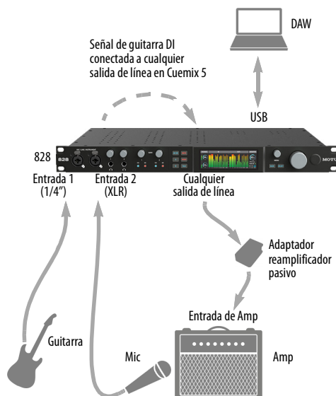
Figura 4-4. Grabación de guitarra para reamplificación.
