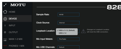
Figura 7-6. Ubicación de Loopback.
