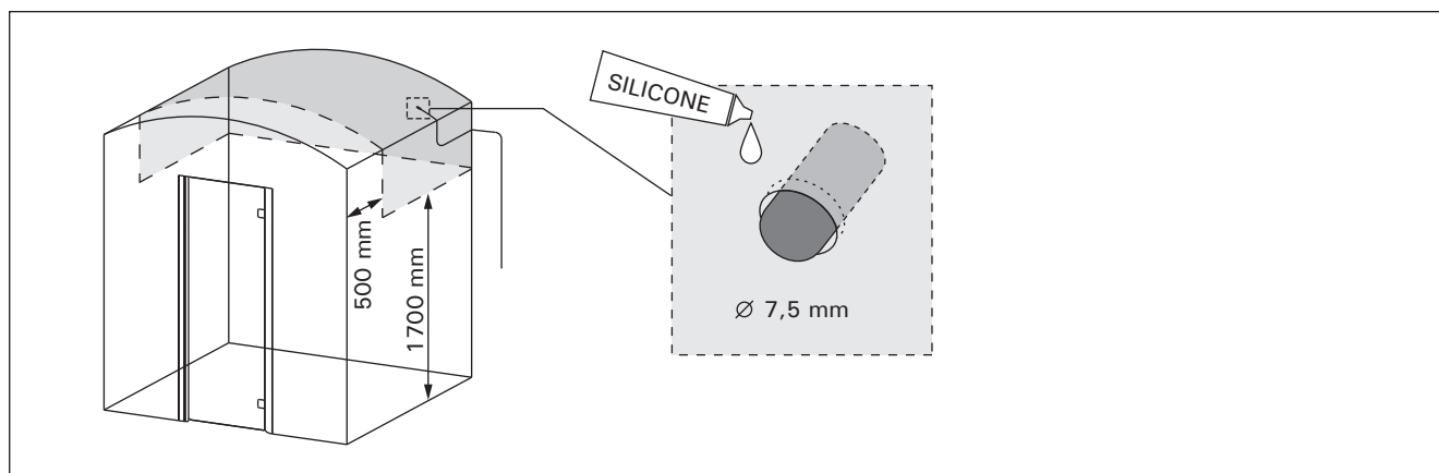
Figura 10. Cómo colocar el sensor de temperatura Figura 10. Posizionamento del sensore di temperatura
