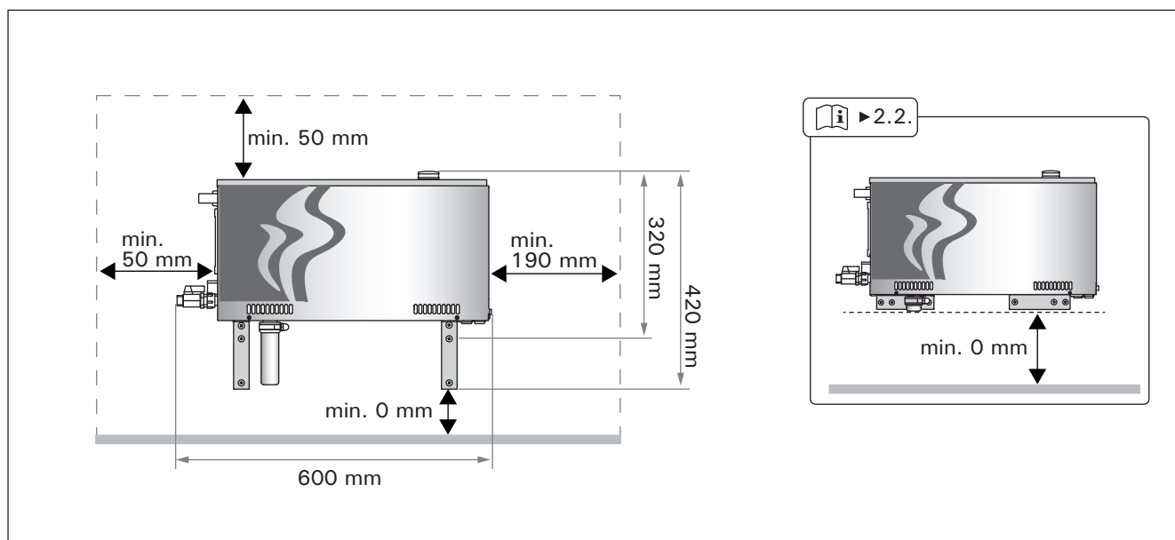
Kuva 5. Asennusmitat Bild 5. Mått vid installation
