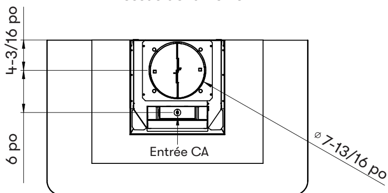
Dessus de la hotte
