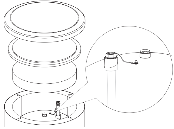
İzole edilmiş koruyucu magnezyum anot.
