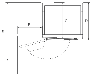
WAND DRAUFSICHT
