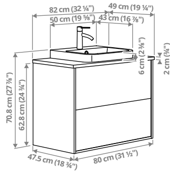
ÄNGSJÖN/エングショーン&BACKSJÖN/バックショーン 洗面台 201 引き出し付き、洗面ボウル、BROGRUND/プログルンド 水栓 82×49×70.8cm
