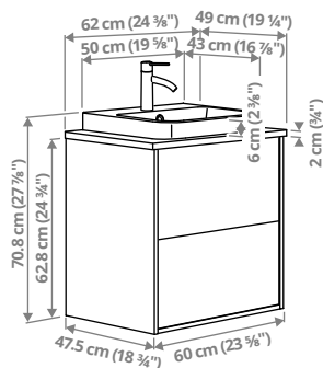
ÄNGSJÖN/エングショーン&BACKSJÖN/バックショーン 洗面台 200 引き出し付き、洗面ボウル、BROGRUND/プログルンド 水栓 62×49×70.8cm
