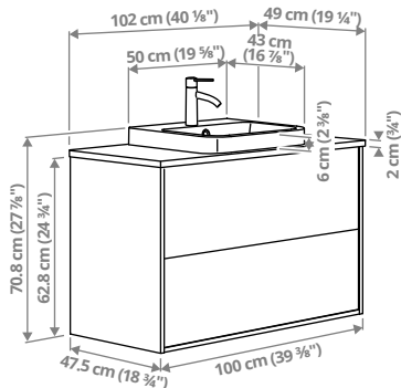
ÄNGSJÖN/エングショーン&BACKSJÖN/バックショーン 洗面台 202 引き出し付き、洗面ボウル、BROGRUND/プログルンド 水栓 102×49×70.8cm
