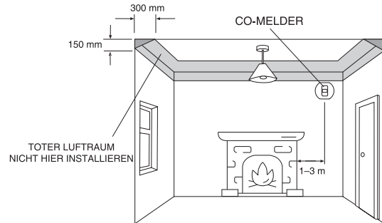
Abbildung 1: Installation in einem Raum mit einem Brennstoffverbrennungsgerät
