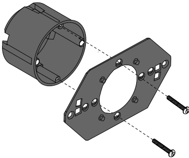
欧盟圆形后箱
