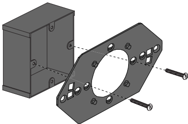
欧盟圆形后箱
