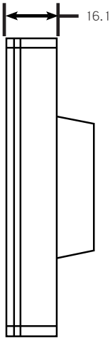
美制 102 mm x 102 mm 接线盒，带单组底圈（水平）
