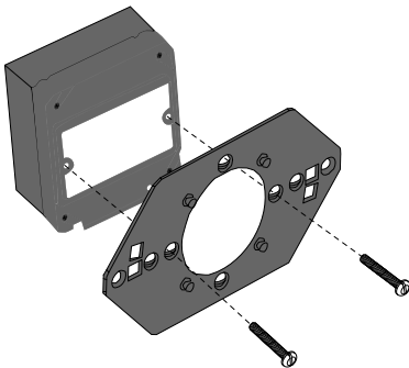
英制方形后箱
