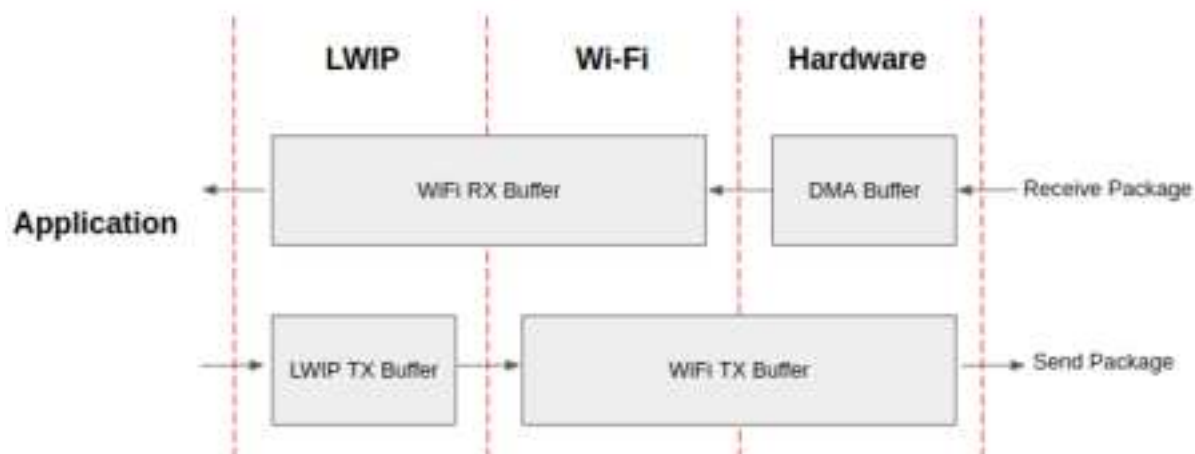
Fig. 84: ESP32 datapath
