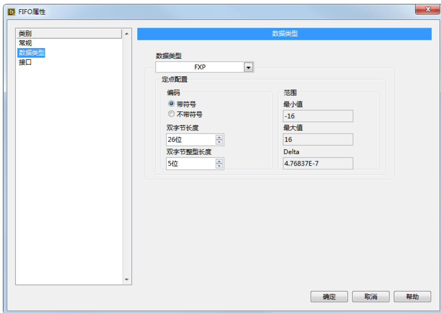
图 8. 配置 DMA FIFO
