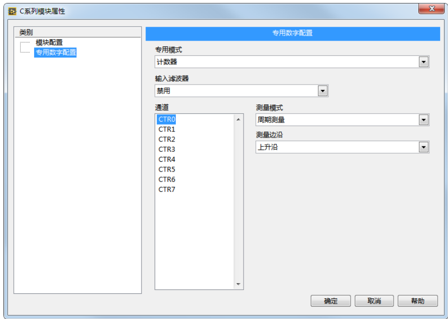
图 6. 配置 DI 模块实现周期测量
