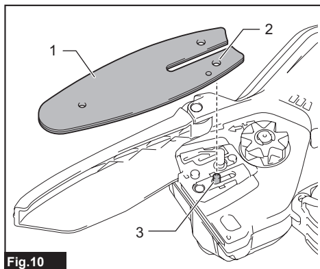
► 1. Guide-chaîne 2. Trou 3. Broche
