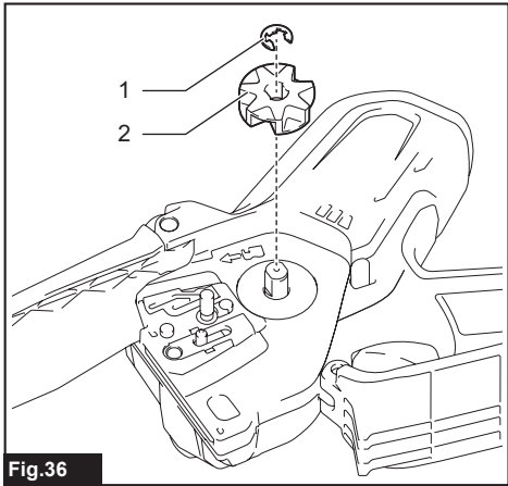
► 1. Anneau de verrouillage 2. Pignon
